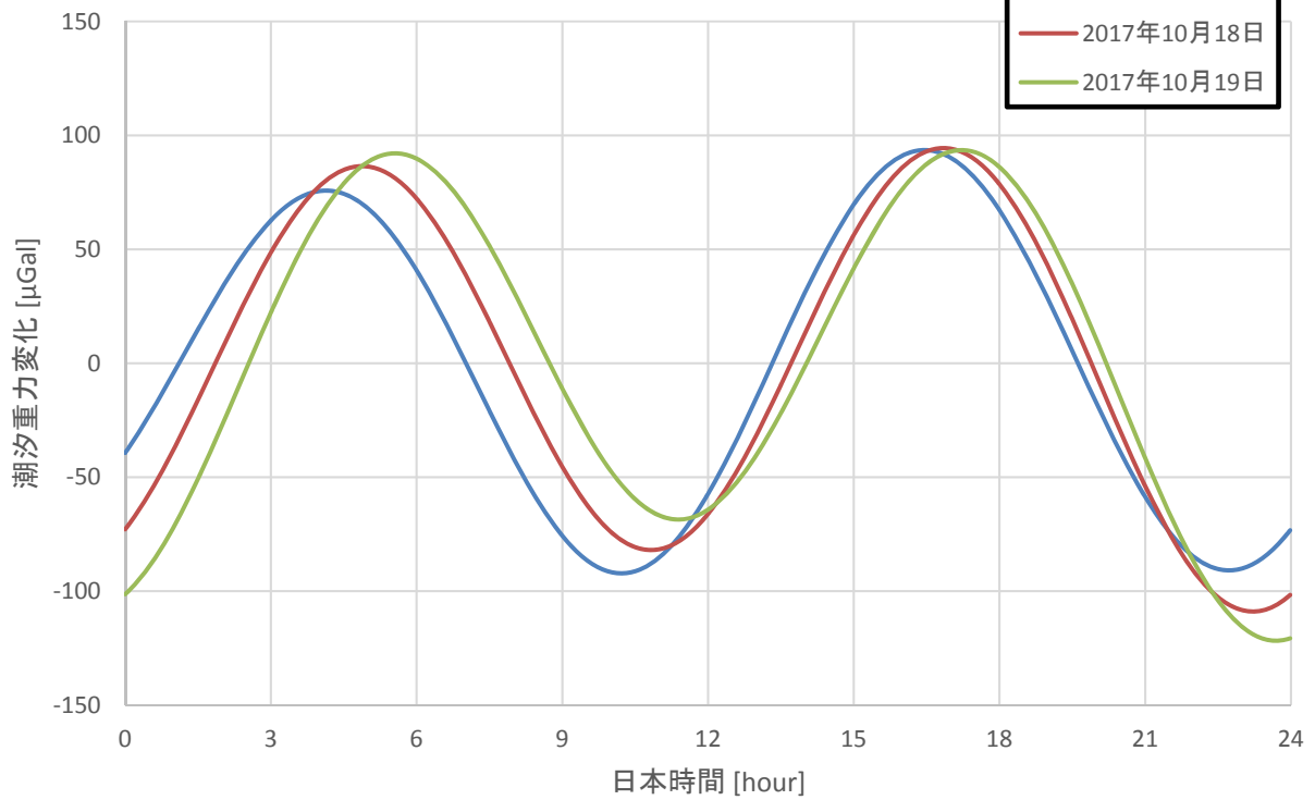
京都の潮汐重力変化(物理量)
